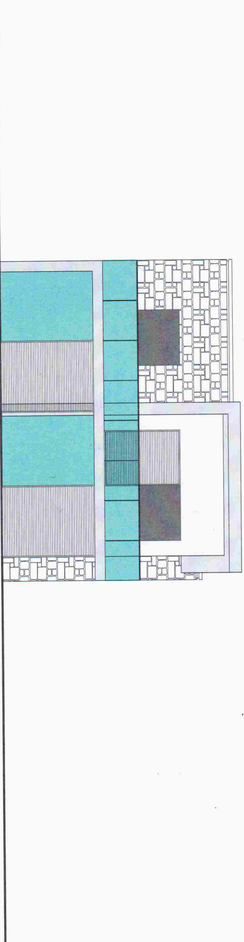
Prospetto sud
